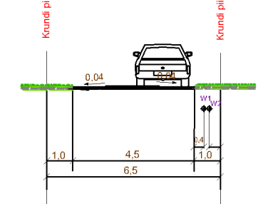
LÕIGE A-A
