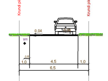
LÕIGE B-B
